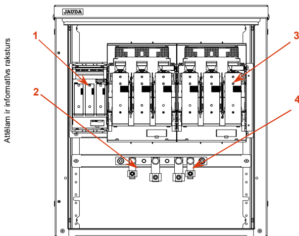
2. att. Aparātūras un elementu izvietojums
