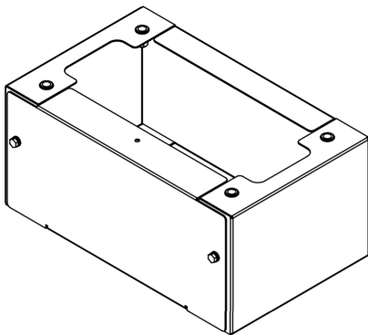
3. att. Cokols C1/170
