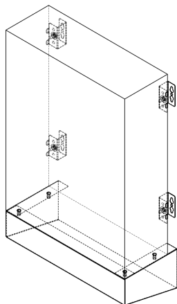
2. att. Kronšteinu komplekts PB-2
