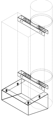
1. att. Kronšteinu komplekts PB-1
