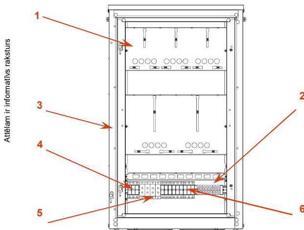
2. att. Aparatūras un elementu izvietojums
