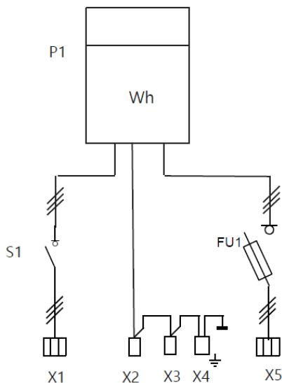
1. att. Elektriskā principshēma
